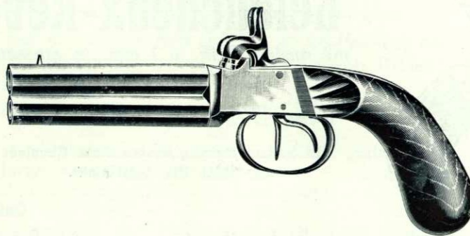
No. 3 kantige Läufe, runder Schaft.
